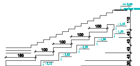
Fundamenty schodkowe
